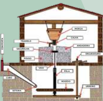
Esquema de um Moinho de Rodízio
